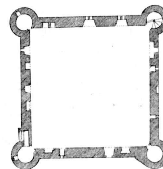
Fig. 310. De Eerste verdieping.
