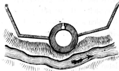
Fig. 88. Toren van Alluye.
