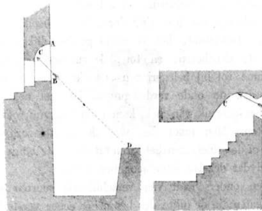
Fig. 81. Doorsnede van een schietgat.
