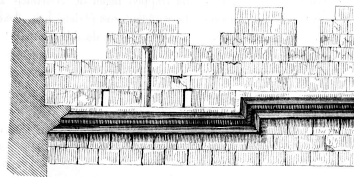
Fig. 76. Courtine van het Kasteel van Beaucaire.
