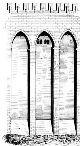
Fig. 62. Machicoulis van het Kasteel der Pausen te Avignon.
