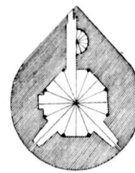
Fig. 45. Platte grond van den Witten Toren te Issoudun.
