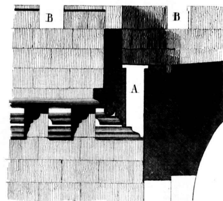
Fig. 61. Machicoulis der Bastille.
