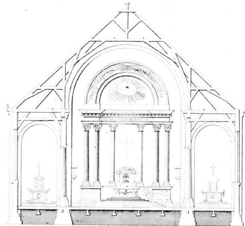
Fig. 2. Doorsnede over de breedte
