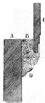
Fig. 60. Doorsnede eener Machicoulis.
