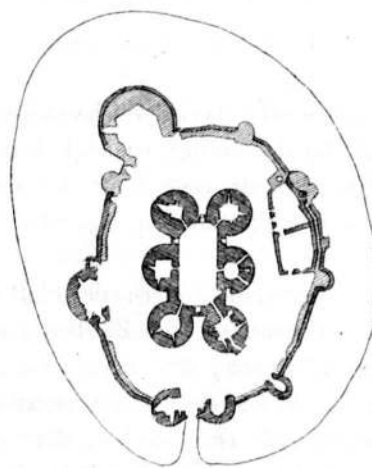
Fig. 83. Plan van het Kasteel te Blanquefort (XIII e Eeuw).
