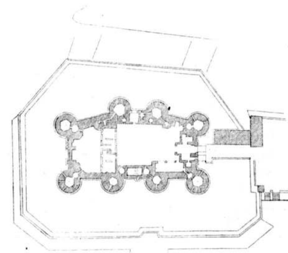
Fig. 304. Plan der Bastille.
